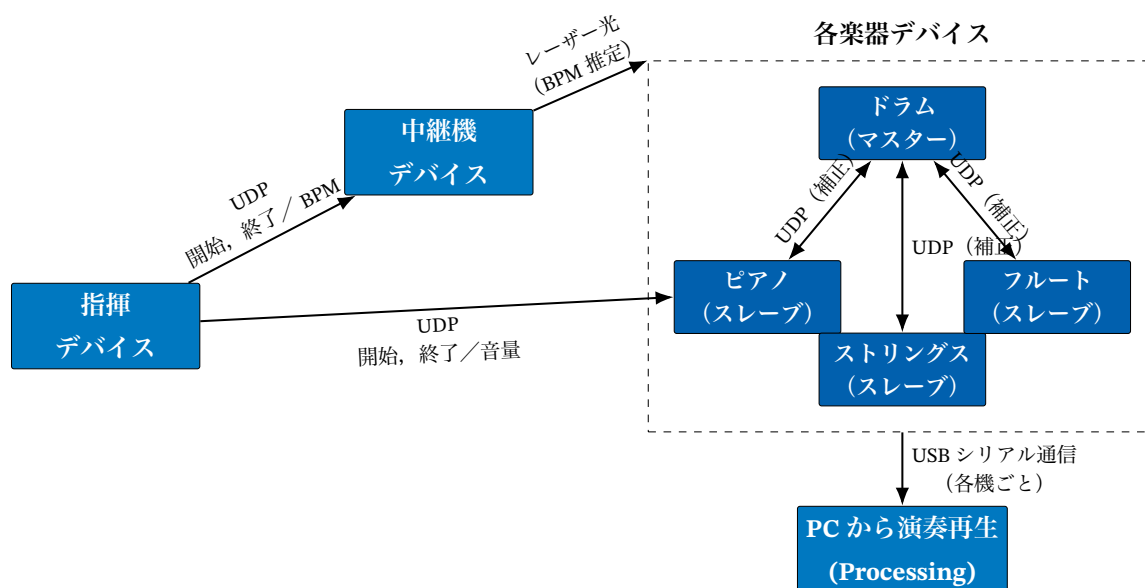
図2 全体の構成図
